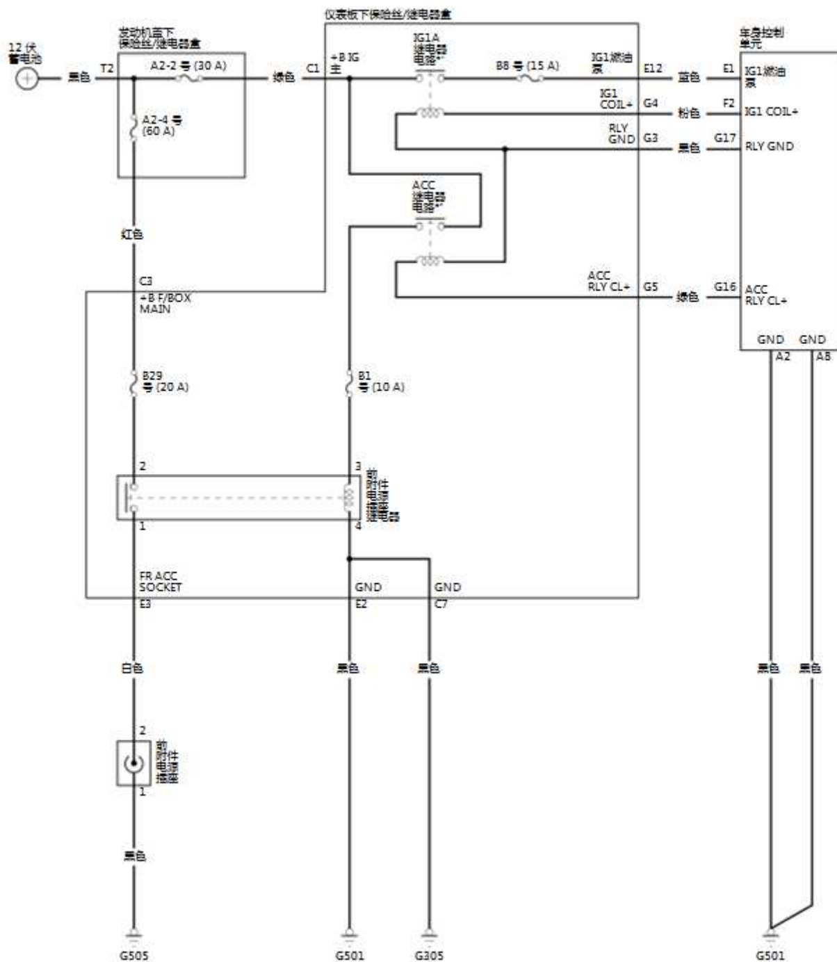
*1:IG1A HOT 处于 ON 和 START 模式 *2:处于 ACCESSORY 和 ON 模式时 ACC HOT
